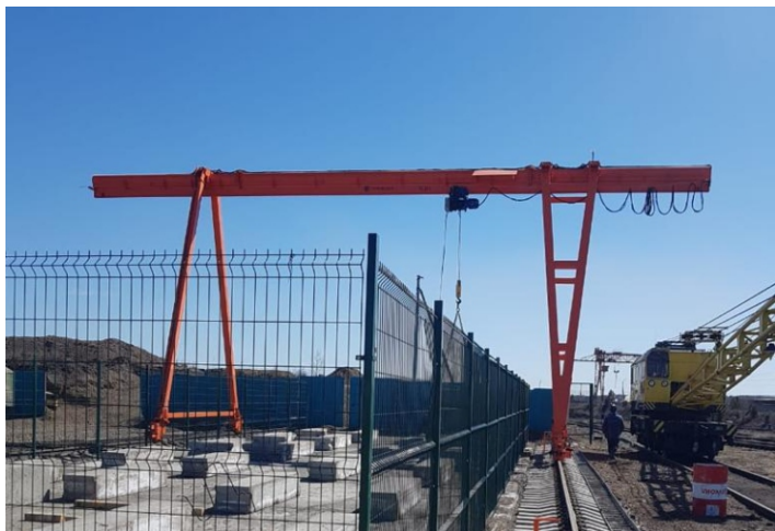
Кран козловой однобалочный с электроприводом грузоподъемностью 10,0 тонн и длиной пролета 19,7 метров для предприятия в поселке Саган-Нур (Республика Бурятия).
